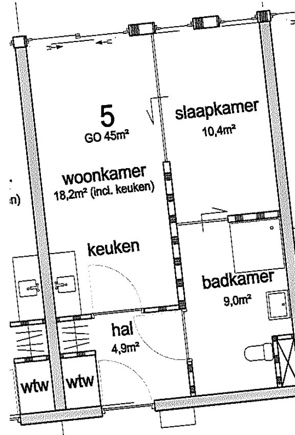
Woningplattegrond Rubenshof, totaal vloeroppervlak 45 m 2
